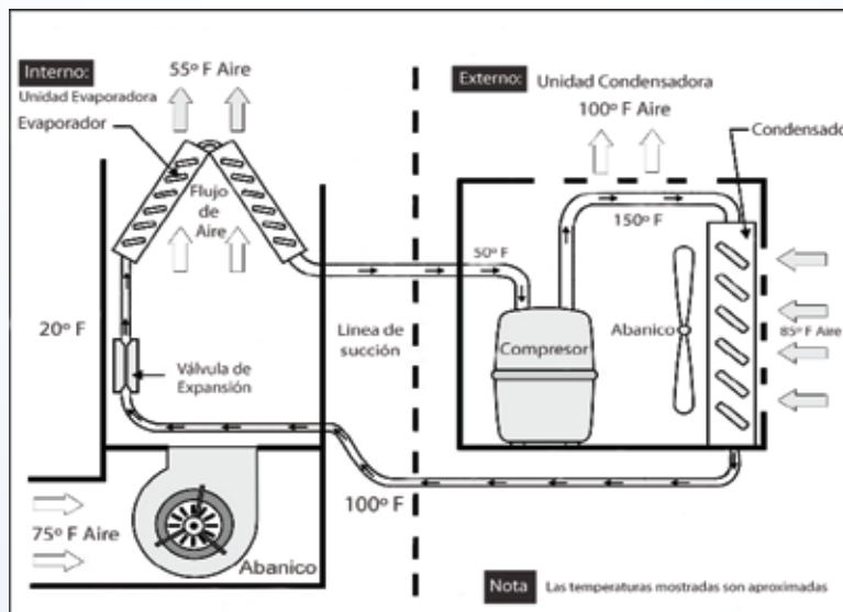
Diagrama 1. Ciclo Básico de Refrigeración
